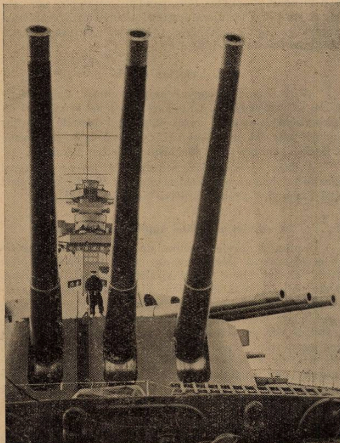
Az angol flotta egyik csatahajójának, a Rodneynek tizenhatcollos óriási ágyú.
